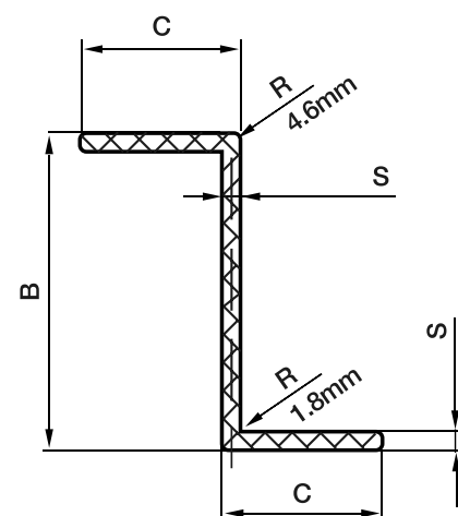
Profil d'ArmaGirt™
